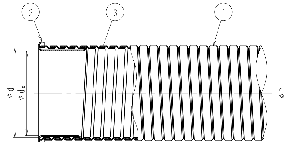
A部詳細図
