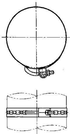
装柱図
