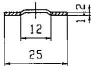
AA断面図
