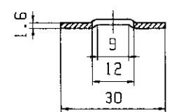
AA断面図
