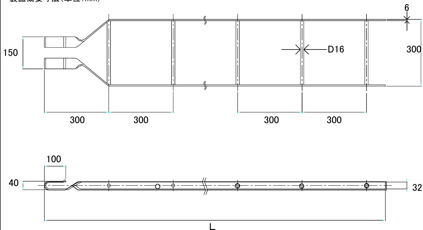
製品概要寸法(単位:mm)
